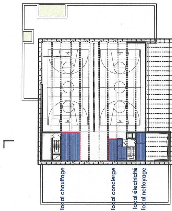
Premier étage 1/500
